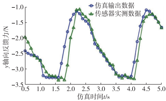
图 11 理论和实测反馈力曲线
