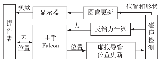
图 1 虚拟力反馈系统框架
