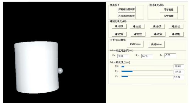
图8 导管末端和血管外壁发生柔性碰撞
