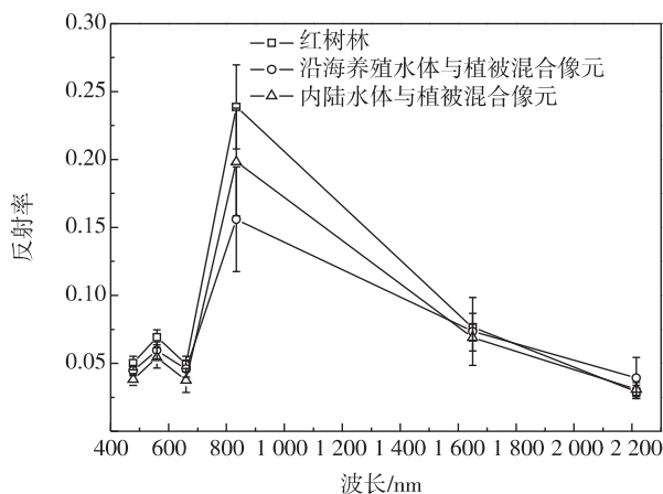
图2 水体与植被混合像元、红树林反射光谱曲线
