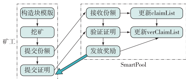
图2 SmartPool 的执行过程
